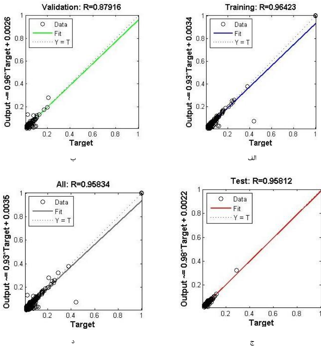
شکل ۶. نمودار برازش و ضریب هم‌بستگی در مراحل مختلف شبکه: الف) مرحله آموزش، ب) مرحله صحت‌سنجی، ج) مرحله آزمون و د) مجموع هر سه مرحله
